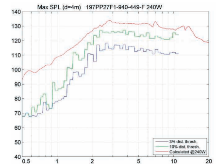
SPLmax 240W - H2 limitiert
