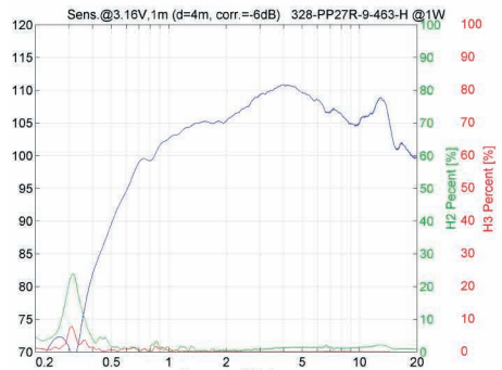
THD 60W - H2 dominiert
