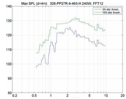
SPLmax 240W - H2 limitiert
