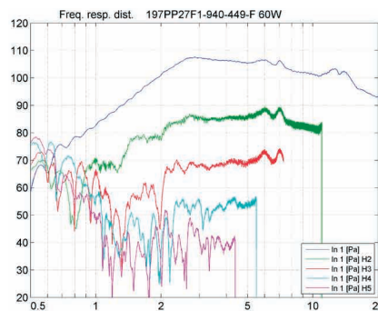
THD 60W - H2 dominiert
